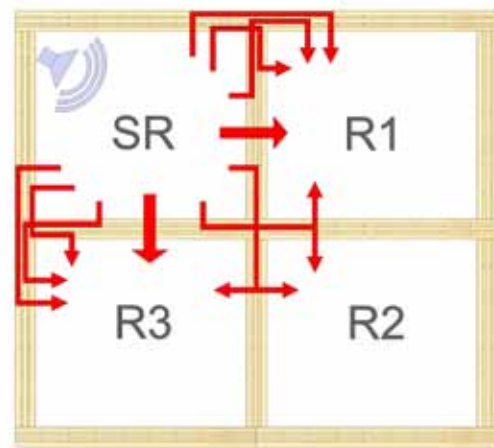
ÜBERTRAGUNGSWEGE LUFTSCHALL
