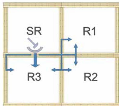
ÜBERTRAGUNGSWEGE KÖRPERSCHALL
