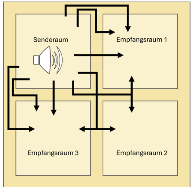
Flanken Luftschall
