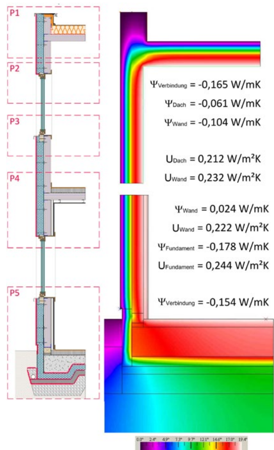
Wärmebrücken Fassade Passivhaus [7.6]
