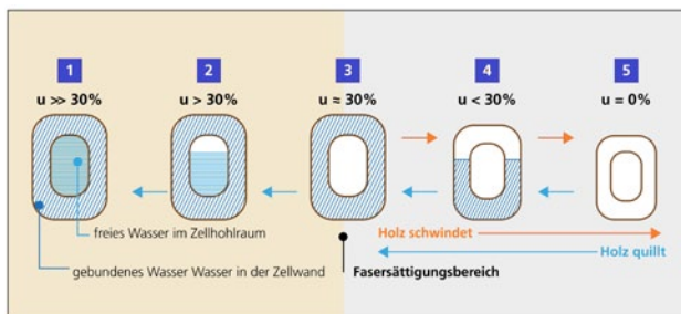
Schemadarstellung Holzzeile [7.3]
