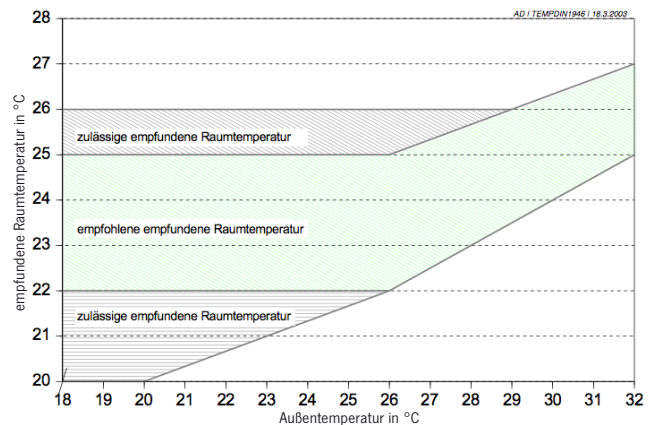
Empfohlene Raumlufttemperatur in Funktion mit der Außentemperatur [7.5]
