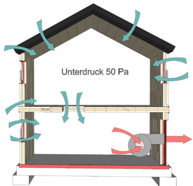
Prinzip Gebäudemessung
