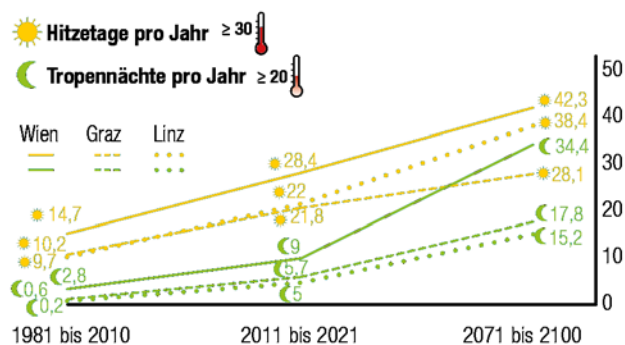
Zunahme der Hitzetage und Tropennächte [7.9]
