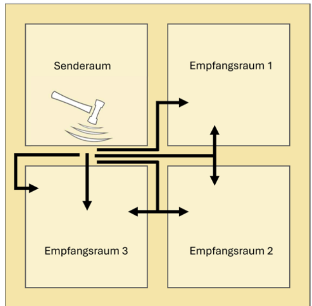
Flanken Trittschall
