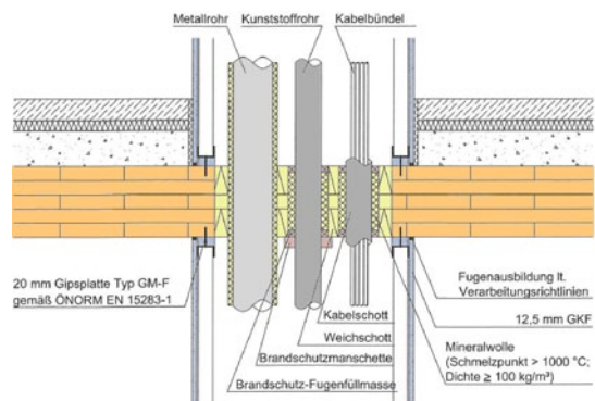
Schachtausführung B; Brandabschottung im Holzbau [7.14]
