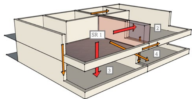
Typische Übertragungsmöglichkeiten in Nachbarräume
