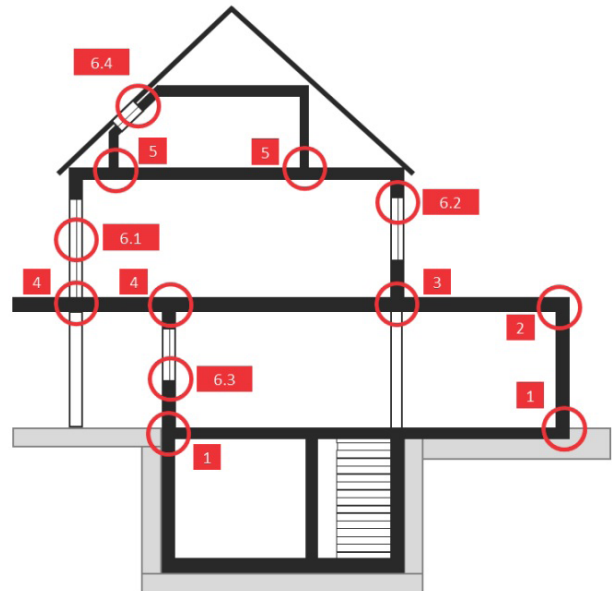
Wärmebrücken Gebäudehülle [7.7]
