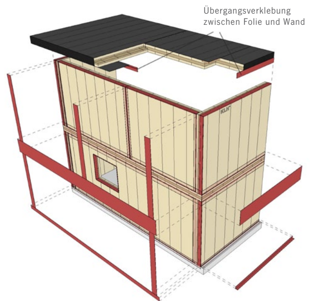
Empfohlene Ausführung ohne vollflächige Folie
