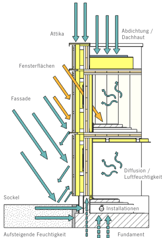
Einwirkungen auf die Fassade
