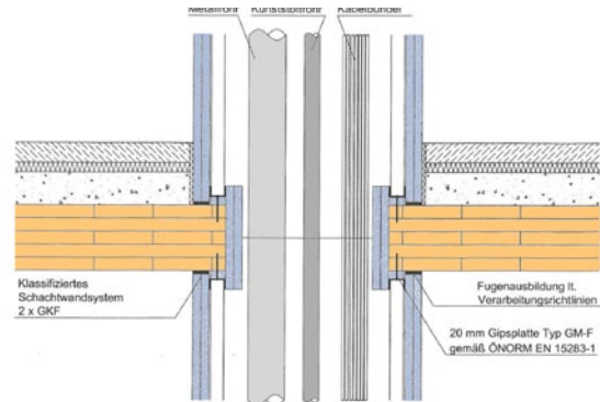
Schachtausführung A; Brandabschottung im Holzbau [7.14]
