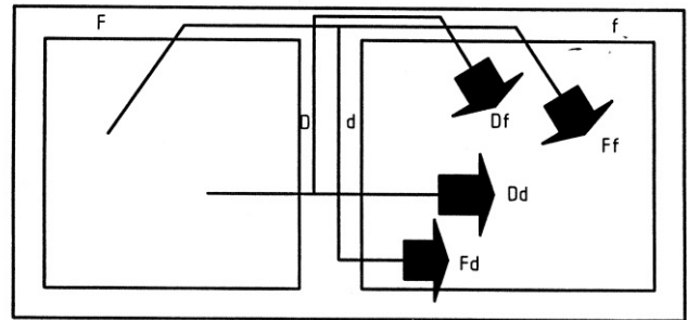
Bezeichnung der Übertragungswege
