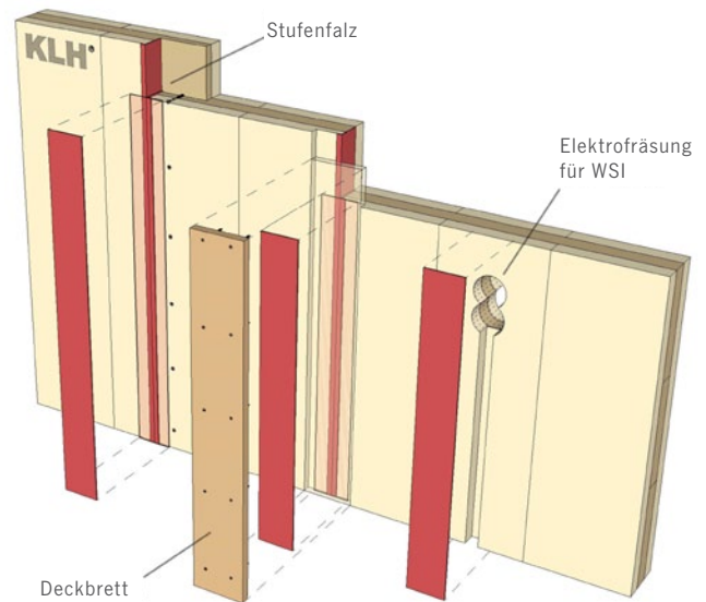
SCHEMA ANSCHLUSSFUGEN
