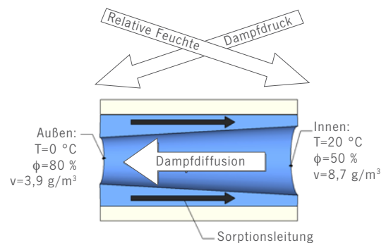
Feuchtetransport im Holz [7.4]
