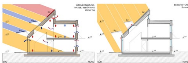
Nutzung der Sonneneinstrahlung, Solaraktivhaus [7.11]
