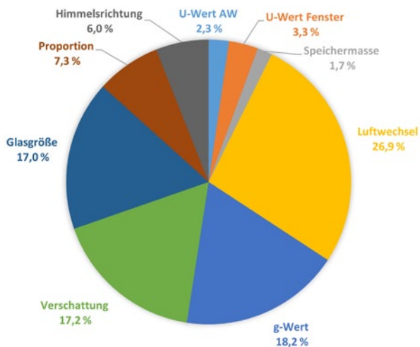
Einflussgrößen sommerliche Überwärmung, Vermeidung von sommerlicher Überwärmung [7.10]
